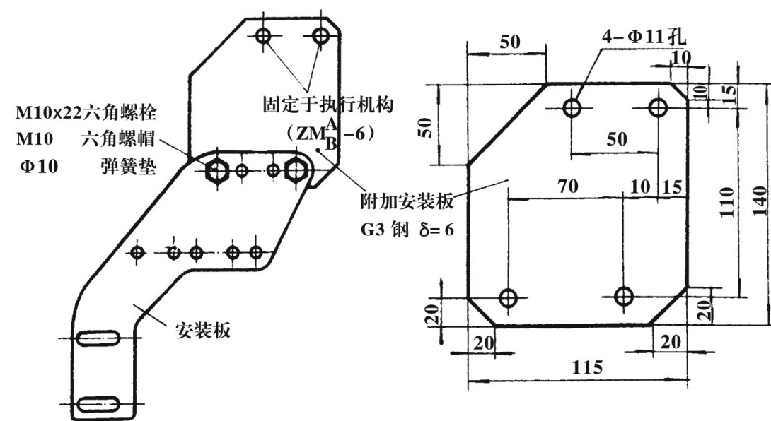
图9 定位器在ZM B A -6型执行机构上用安装板
